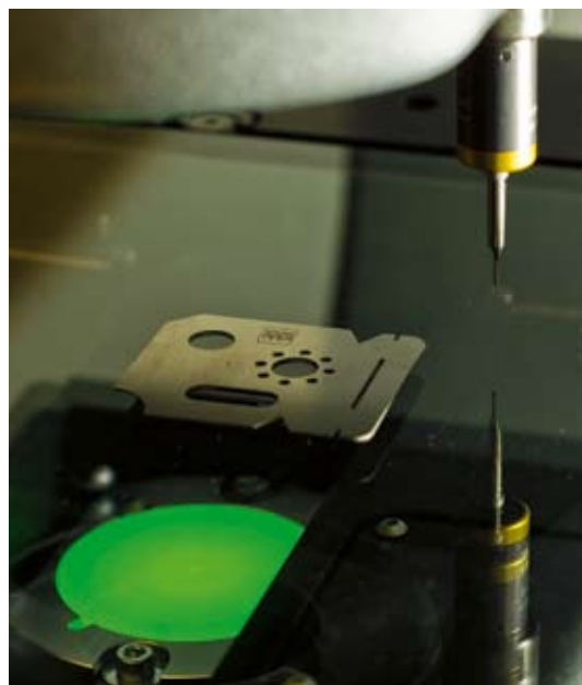
Mätning med optisk mätmaskin av märket Tesa Visio.
