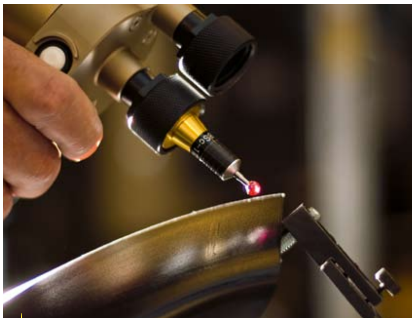
Mätning med mobil mätarm av märket CimCore.
